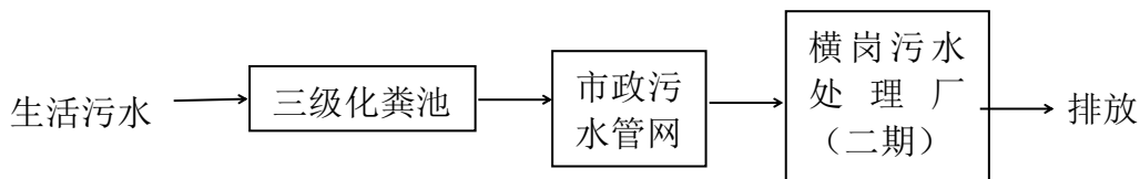
图 8-1 生活污水处理工艺流程图
