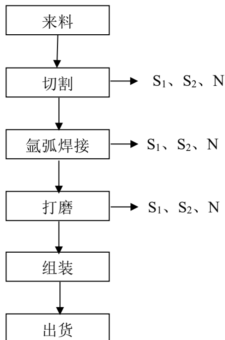
图 6-1 不锈钢厨具工艺流程及产污环节
