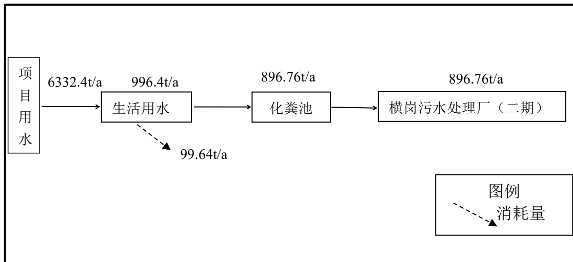
图 6-2 项目水平衡图
