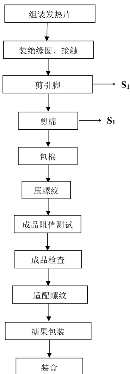
图 5-2 电子烟雾化芯工艺流程及产污环节
