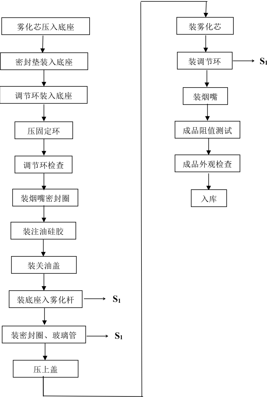
图 5-1 电子雾化器工艺流程及产污环节
