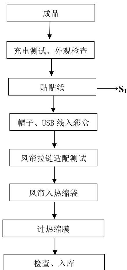
图 5-5 风帘帽工艺流程及产污环节
