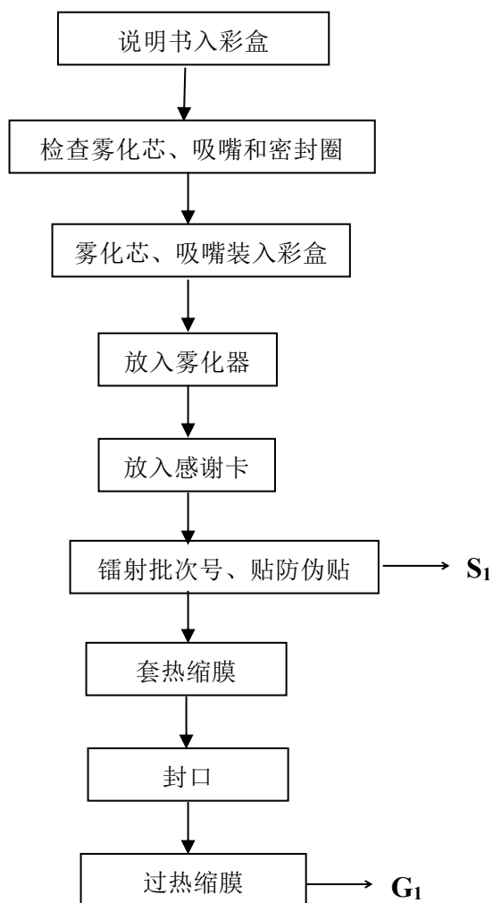
图 5-1 电子雾化器工艺流程及产污环节
