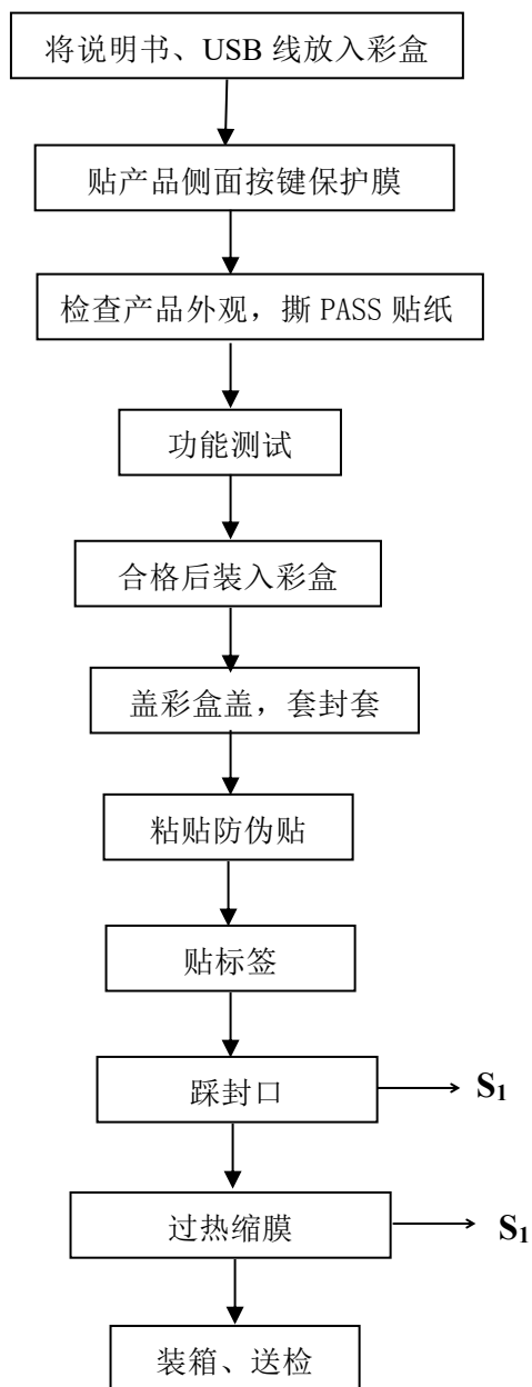
图 5-3 电子烟工艺流程及产污环节
