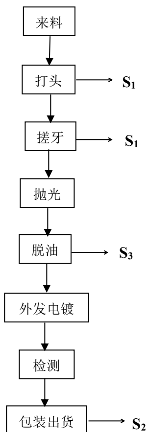
图 5-1 螺丝工艺流程及产污环节
