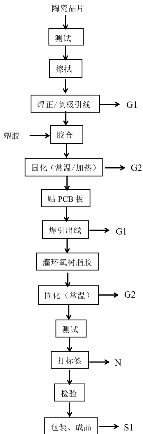
图 5-1 超声波传感器的工艺流程及产污工序
