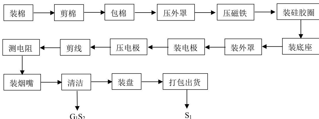
图 5-1 烟弹与雾化芯生产工艺流程图
