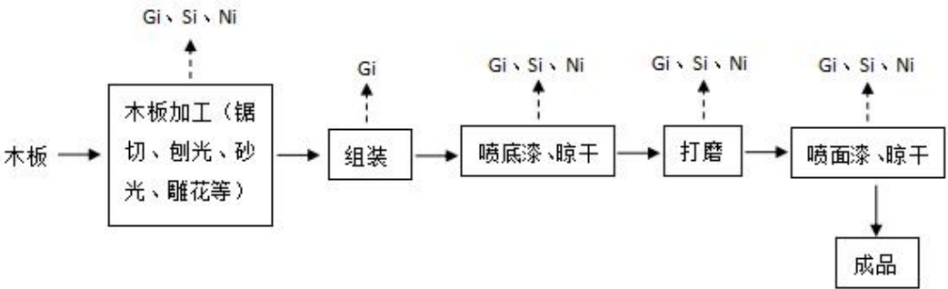
图 2-1 木质家具运营期工艺流程及产污环节图
