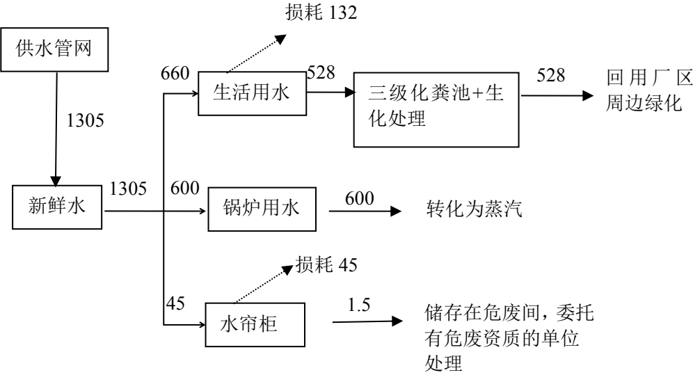
图 2-1 项目给排水平衡图 (t/a)
