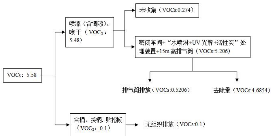
图 2-1 项目 VOCs 物料平衡图 (t/a)
