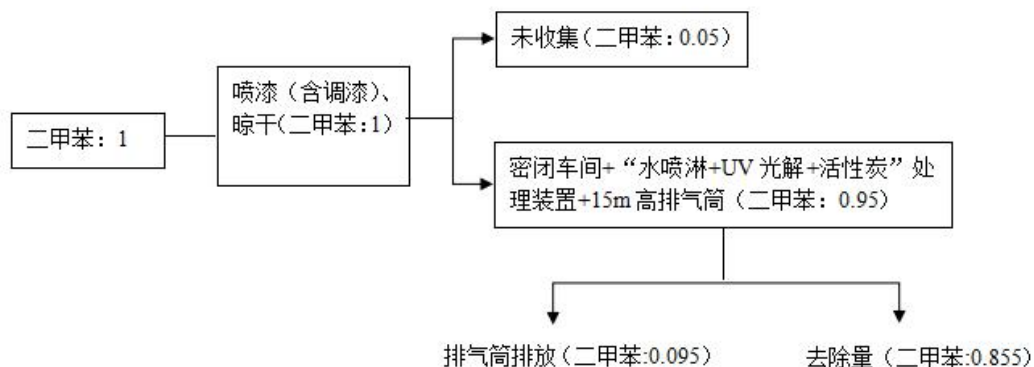
图 2-2 项目二甲苯物料平衡图 (t/a)
