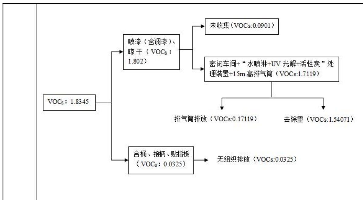
图 2-1 项目 VOCs 物料平衡图 (t/a)
