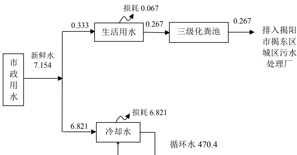
图 2-1 项目给排水平衡图 (t/d)
