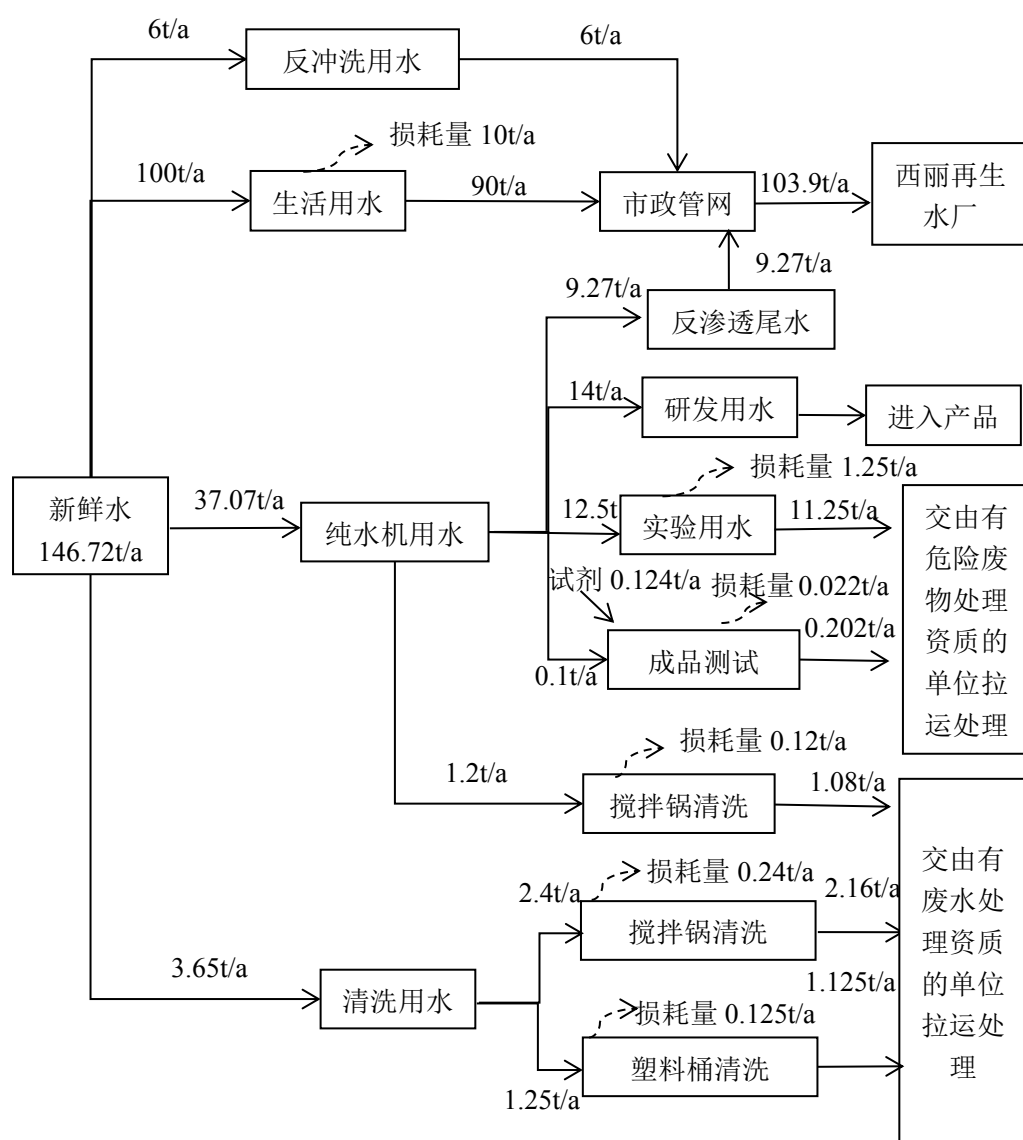
图 2-2 项目改扩建后水平衡图
