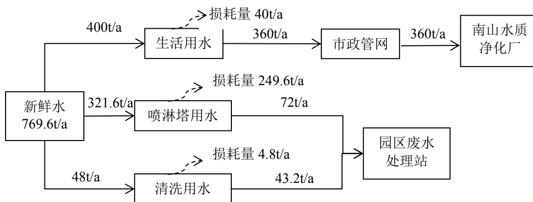
图 2-2 项目扩建后水平衡图
